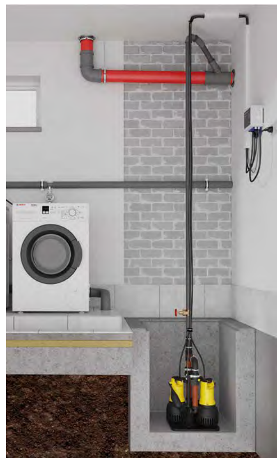
Schmutzwasserpumpen einfach und schnell installiert. Hier eine Doppelanlage mit EASYFIX 32 Duo. Die zugehörige Steuerung regelt das Zusammenspiel beider Pumpen
